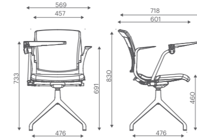
Myko Base Swivel Glide 4-M8PL-M013-M054-M402-A
